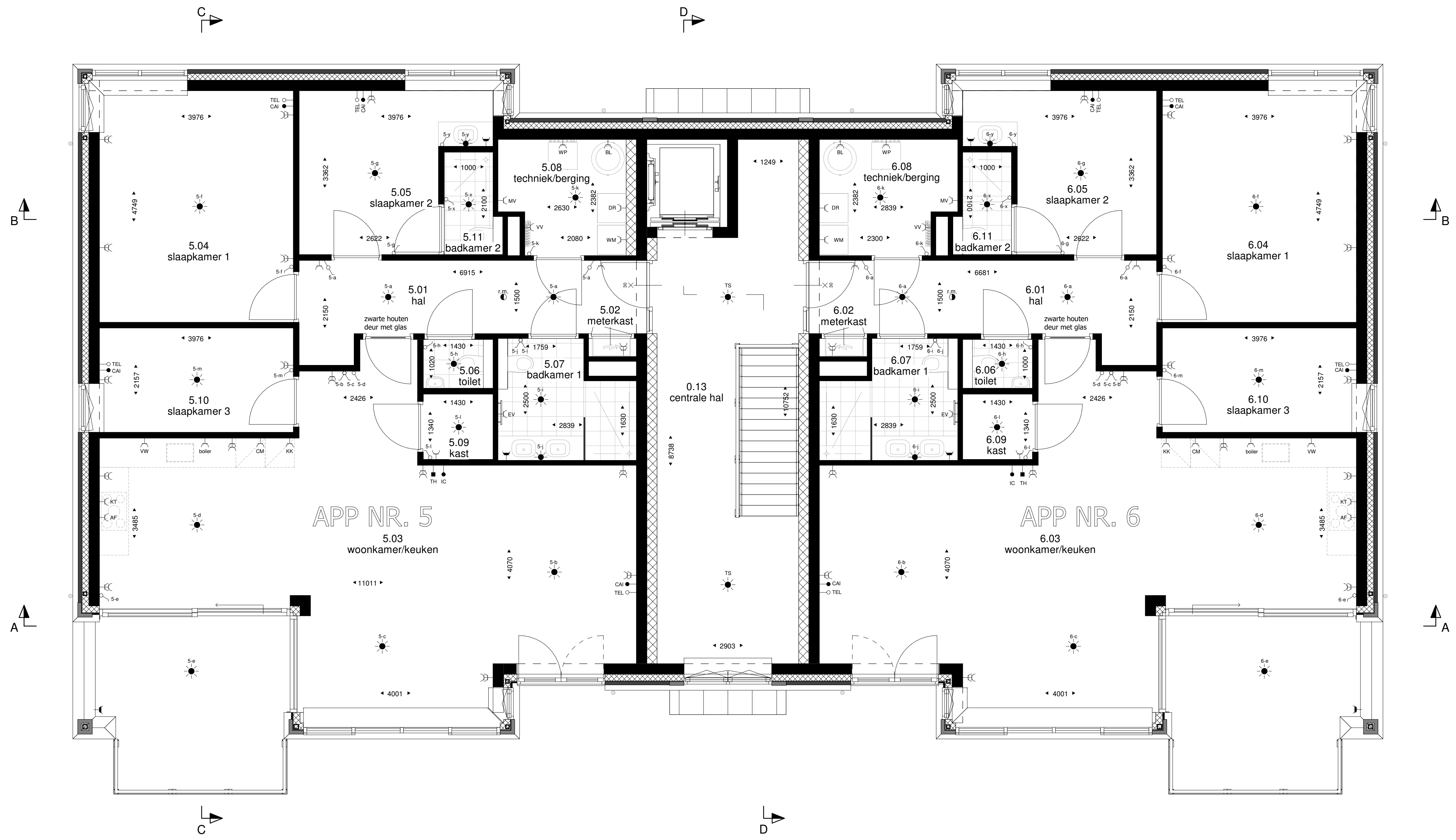
2e VERDIEPING 1 : 50
