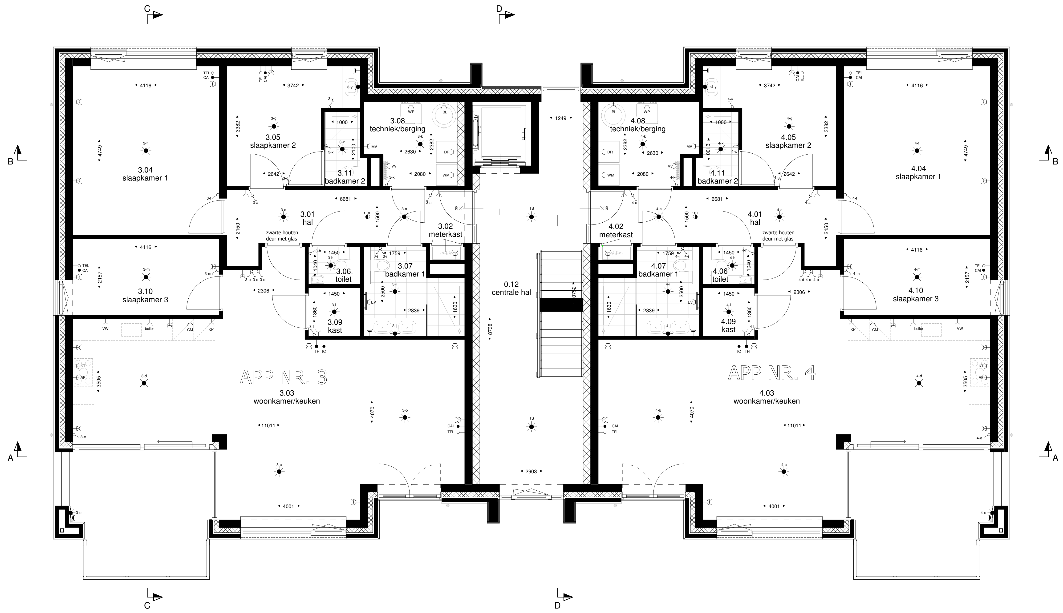
1e VERDIEPING 1 : 50
